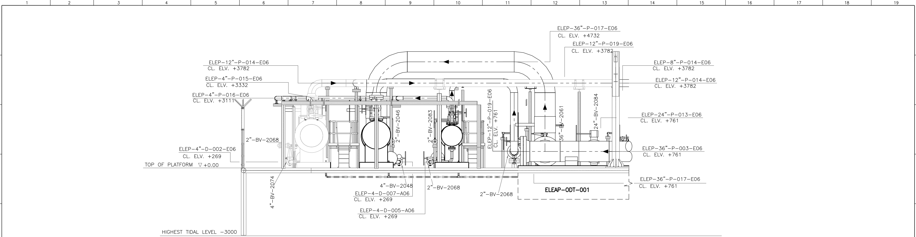
A 01 SECTION A-A
